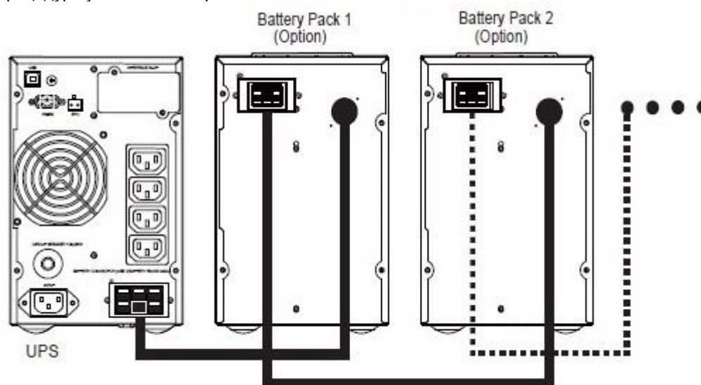
Рис. 3. Пример подключения внешнего батарейного блока к ИБП
