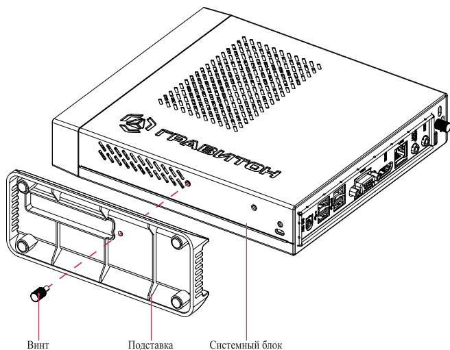
Рисунок 2 – Установка ПК «Гравитон» на подставку
