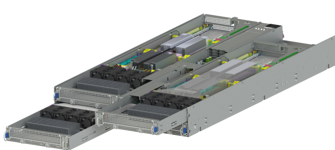
Сервер ПАЛАДИН-МШУ (тип 3) / Вид спереди без верхней крышки
